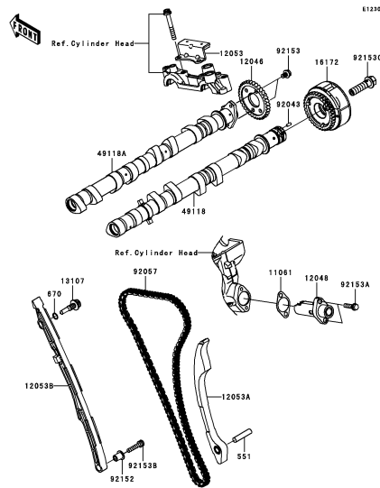
B-10 Camshaft(s)/Tensioner
