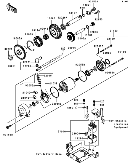
D-4 Starter Motor
